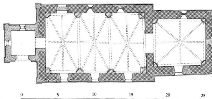
Fig. 5. Grundplan 1:300, tegnet af KdeFL 1990 efter Aksel Skov 1964. Størrelse og nærmere placering af \uparrow våbenhus (s. 3575) på kirkens sydside kendes ikke. – Ground-plan.
