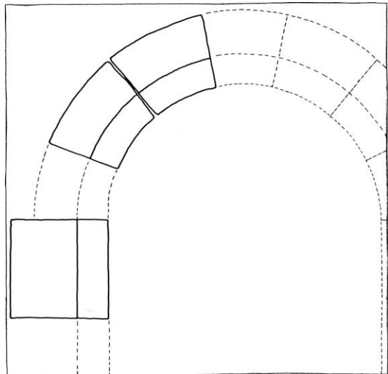
Fig. 11. Skematisk forslag til anbringelse af de tre profilerede *hjørnekvadre (s. 3573, jfr. fig. 10), 1:25. KdeFL 1990. - Suggested position of the moulded ashlars, cf. fig. 10.
