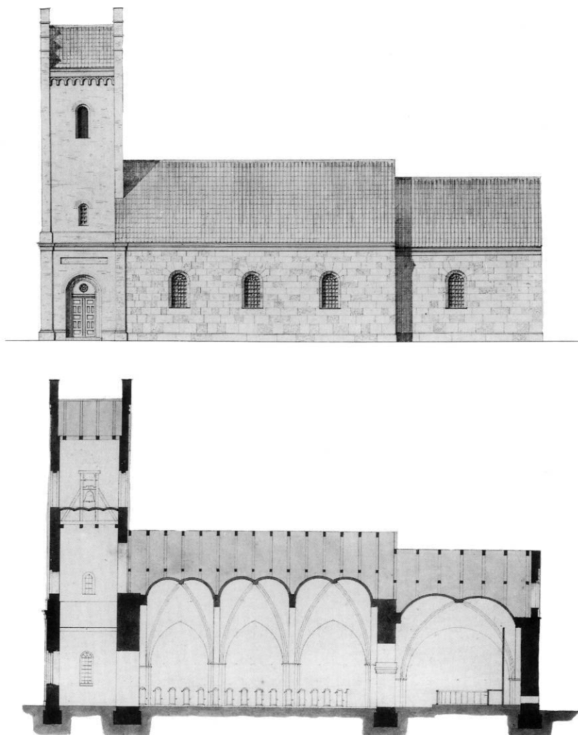
Fig. 4. Sydfacade og længdesnit 1:300, tegnet af Carl Kiilsgaard 1890. Frijsenborg godsarkiv, Hammel. – Elevation of the south side and longitudinal section.
